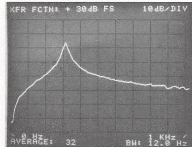
b) Random noise stimulus
