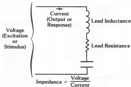
a) Actual impedance of a real capacitor
